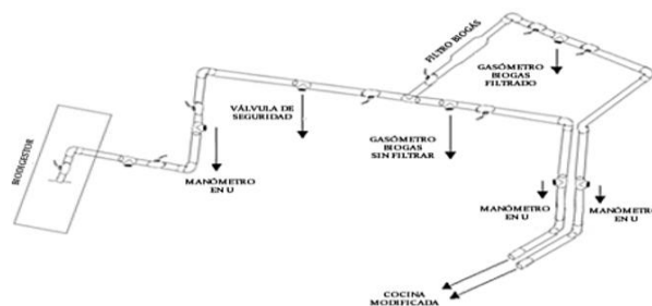
Figura 5. Esquema de la trayectoria del biogás
