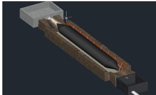
Figura 1. Diseño del biodigestor en AUTOCAD
