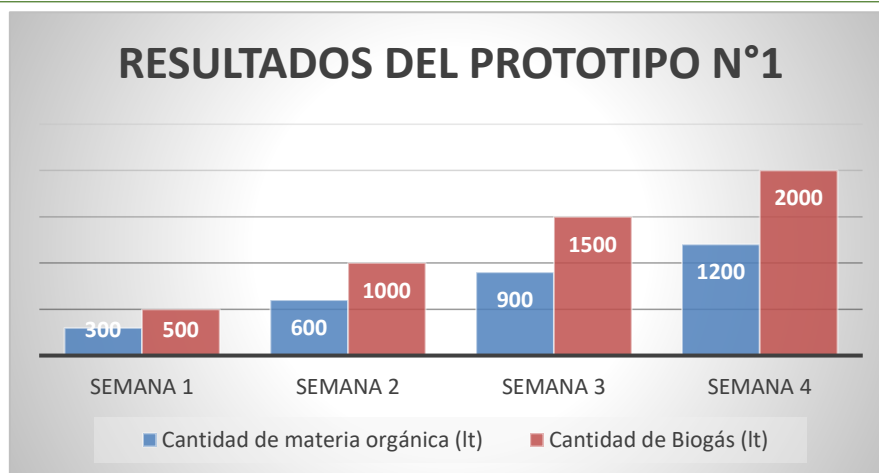
Gráfico 1. Cantidad de biogás según la cantidad de materia orgánica en un determinado tiempo
