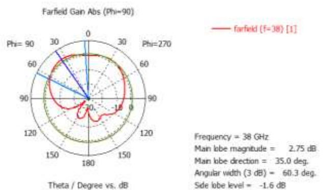
Gambar 8. Pola Radiasi Frekuensi 38 GHz
