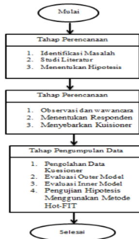
Gambar 1. Metodologi Penelitian
