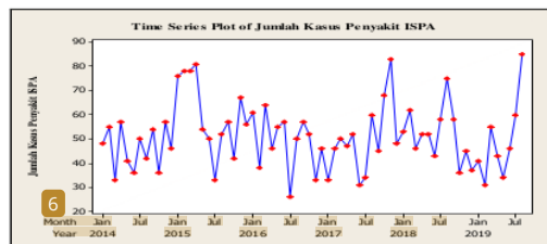
Gambar 1. Plot Data Aktual Kasus ISPA
