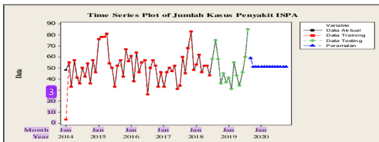
Gambar 6. Grafik Peramalan Jumlah Kasus Penyakit ISPA
