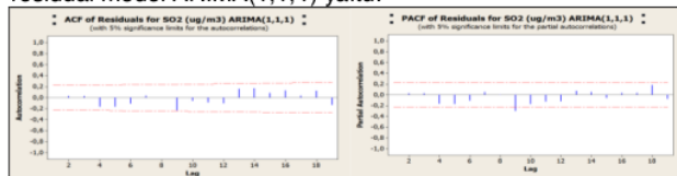
Gambar 6. Plot ACF dan PACF bagi Residual Model ARIMA(1,1,1)
