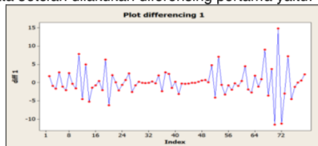
Gambar 4. Plot Data Sulfur Dioksida ( \text{SO}_2 ) setelah Differensing Pertama
