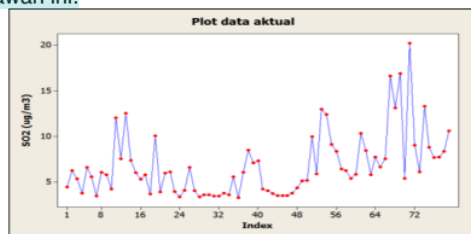
Gambar 2. Plot Data Aktual Kepekatan Sulfur Dioksida ( \text{SO}_2 )
