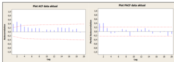
Gambar 3. Plot ACF dan PACF Data Sulfur Dioksida ( \text{SO}_2 )
