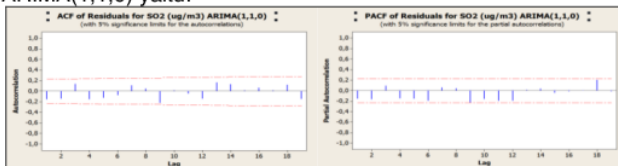
Gambar 8. Plot ACF dan PACF bagi Residual Model ARIMA(1,1,0)
