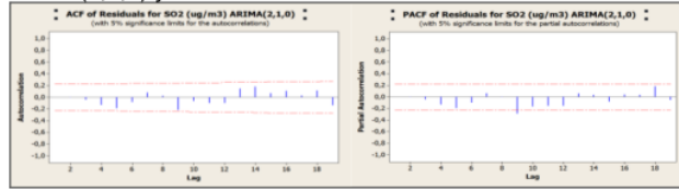
Gambar 9. Plot ACF dan PACF bagi Residual Model ARIMA(2,1,0)
