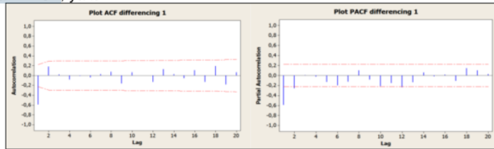
Gambar 5. Plot ACF dan PACF Data Sulfur Dioksida (SO 2 ) setelah Differensing Pertama
