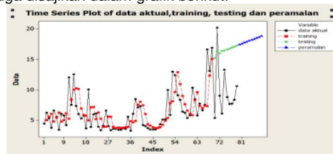
Gambar 10. Grafik Peramalan training , Testing dan Peramalan Kepekatan Sulfur Dioksida
