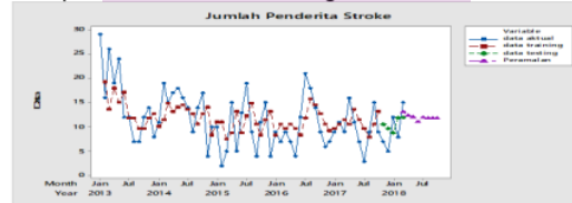
Gambar 6. Grafik Peramalan Training , Testing dan Peramalan Tahun 2018
