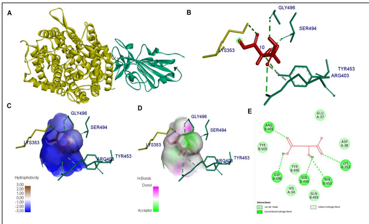
Gambar 2. A dan B Interaksi antara senyawa asam malat dan kompleks protein spike glycoprotein – ACE2. C struktur 3D kompleks antara asam malat dan spike glycoprotein – ACE2. D profil hidrofobisitas kompleks. E profil ikatan hidrogen kompleks senyawa dan spike glycoprotein – ACE2, E. struktur 2D kompleks senyawa dan spike glycoprotein – ACE2.
