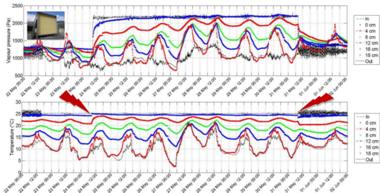
Figure 4. Evolution des pressions partielles de vapeur et des températures à différentes profondeurs dans la paroi n°3 (16cm de fibre de bois + enduit extérieur) sur la cellule Passys, soumise au climat naturel à l'extérieur et à un échelon d'humidité à l'intérieur.
