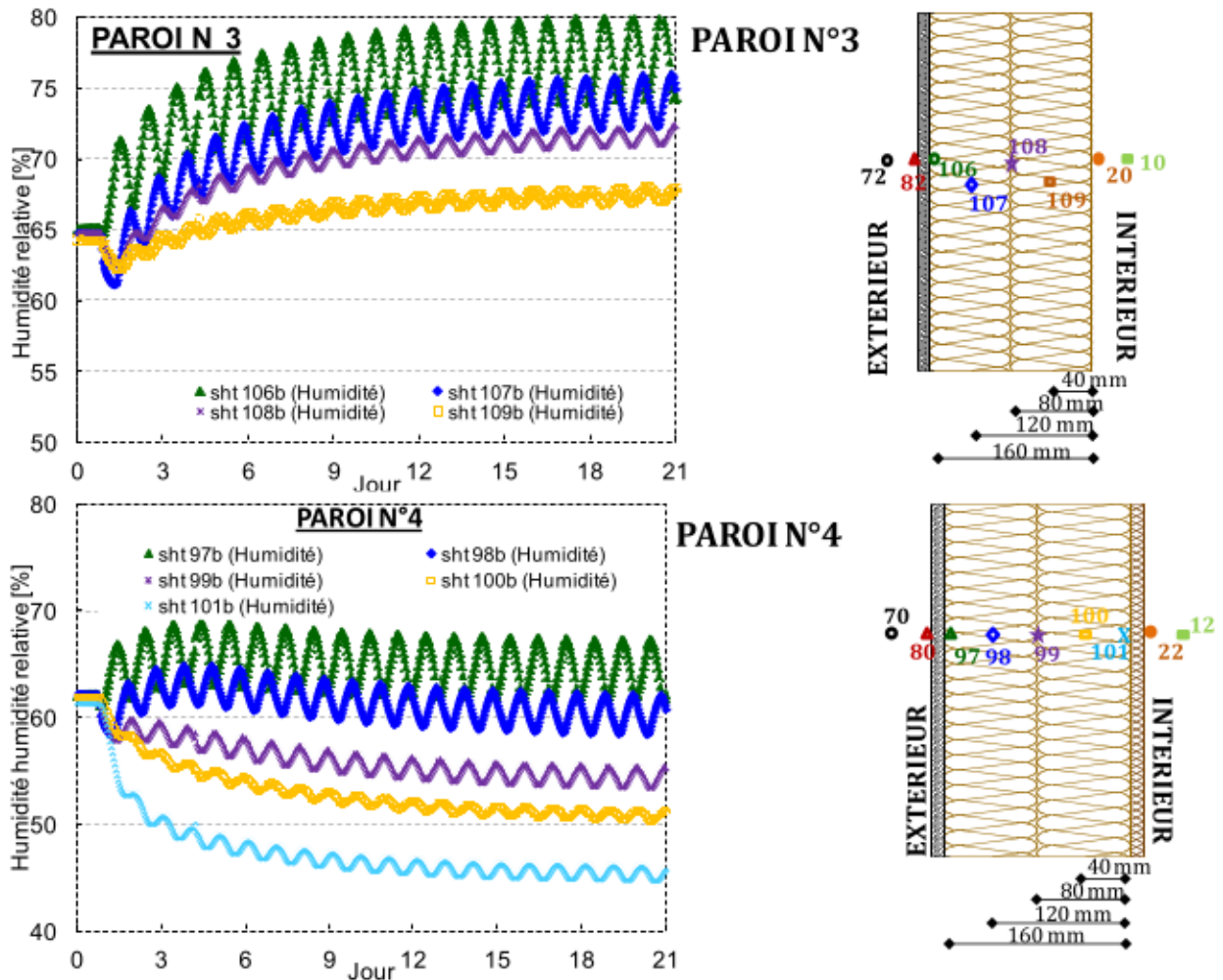
Figure 3. Evolution temporelle des profils de température et d'humidité relative de l'air dans les parois avec la fibre de bois seule (N° 2), protégé par l'enduit extérieur(N°3) et protégé par l'enduit extérieur et OSB (N°4), soumise à des conditions climatiques oscillantes.
