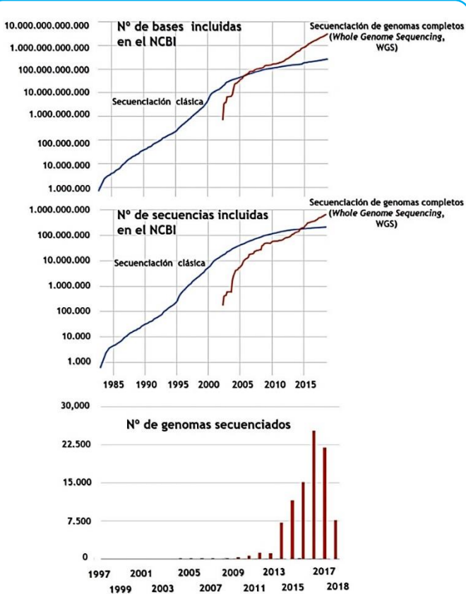
Figura 2 Evolución del número de bases y secuencias incluidas en la base de datos NCBI (National Center of Biotechnology Information) del Instituto Nacional de Salud de EEUU [11] y del número de especies secuenciadas según el Genome Online Database (GOLD) [12].
