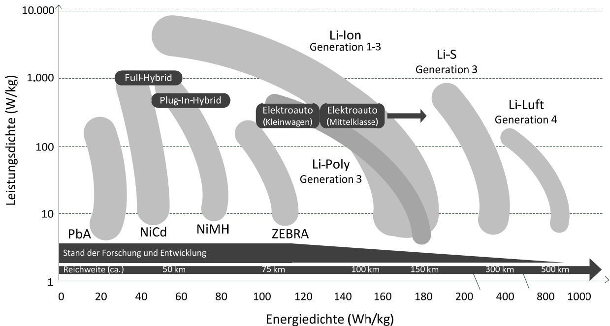
Abb. 8: Energie- und Leistungsdichten der Batterietechnologien für automobilen Anwendungen [eigene Darstellung in Anlehnung an Kalh07, S.25 und Npez11, S.19]
