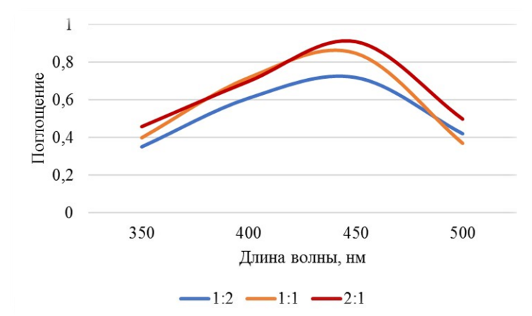
Рис. 3. Спектр поглощения золь наночастиц серебра, полученных использованием экстракта хвойных опилок и \text{AgNO}_3 в разном соотношении
