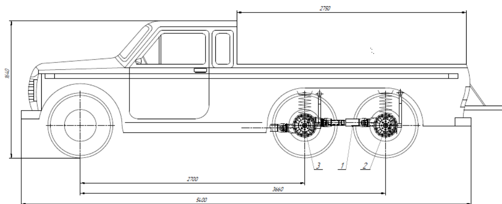
Рис. 1. Эскиз трехосной машины
