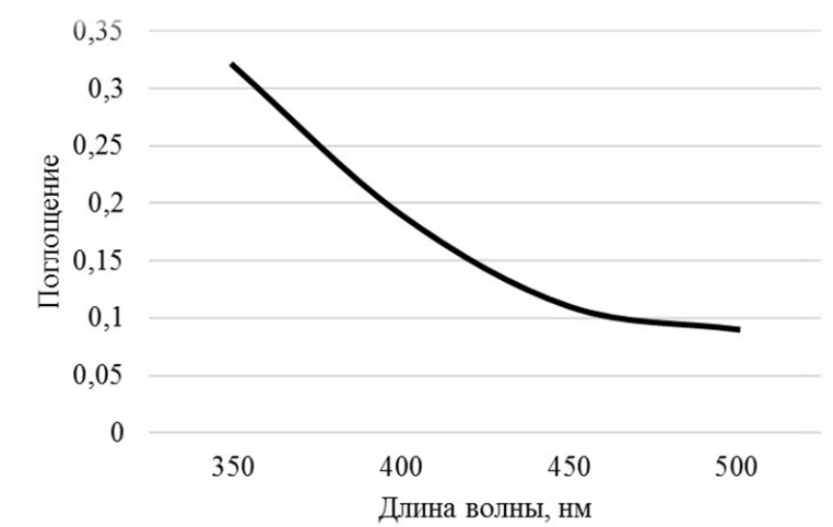
Рис. 2. Спектр поглощения экстракта хвойных опилок
