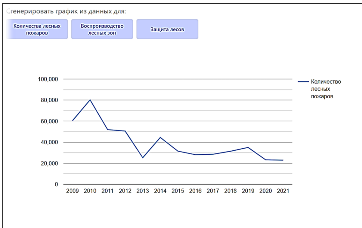
Рис. 2. Созданное web-приложение
