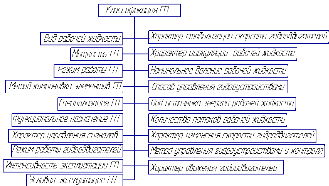
Рис. 4. Классификация гидроприводов
