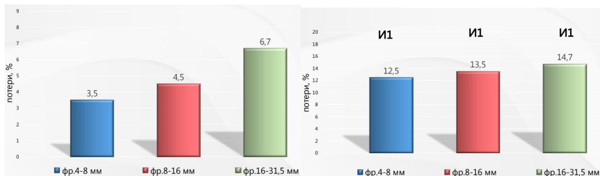
Рис. 2. Показатели дробимости и истираемости щебня Баженовского месторождения различных фракций в процентах
