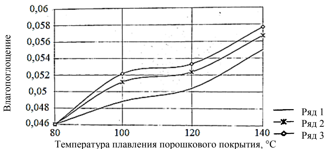
Рис. 2. Зависимость влагопоглощения от температуры плавления эпоксидно-полиэфирного порошкового покрытия при различном времени отверждения Ряды 1, 2, 3 – 4, 6, 8 минут, соответственно
