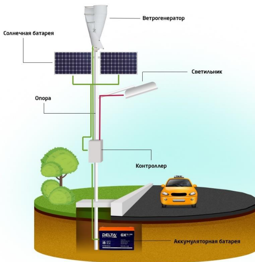
Рис. 1. Схема уличного освещения на солнечной батарее и ветрогенераторе
