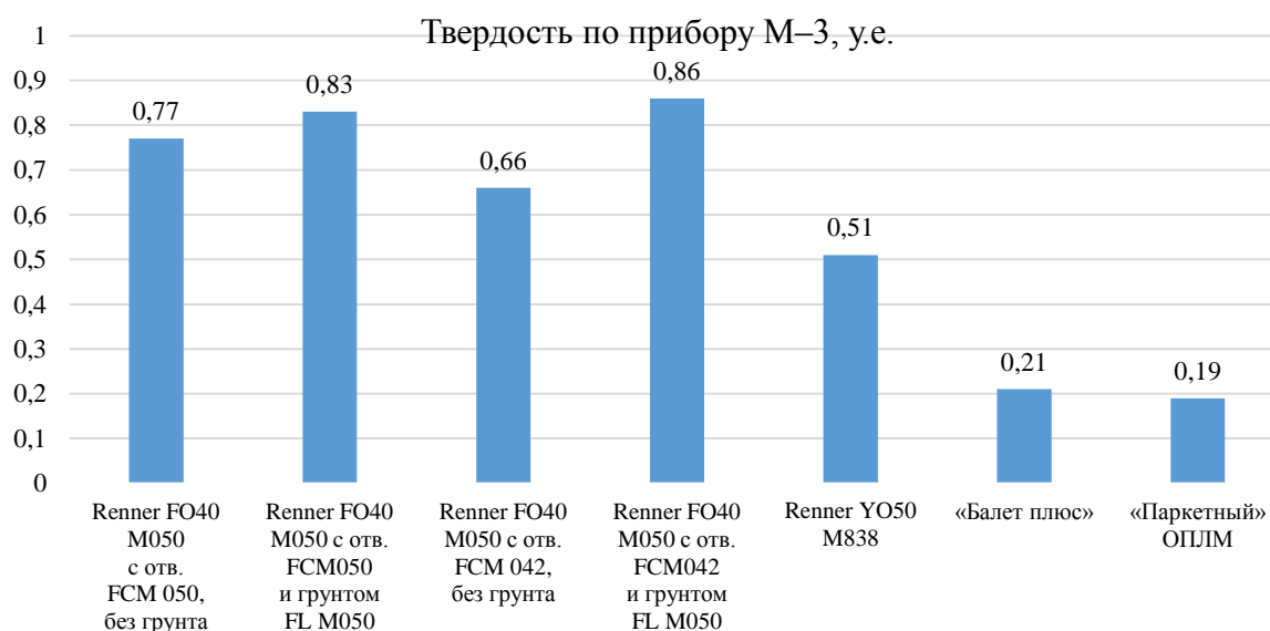
Рис. 2. Результаты испытаний твердости по прибору М-3
