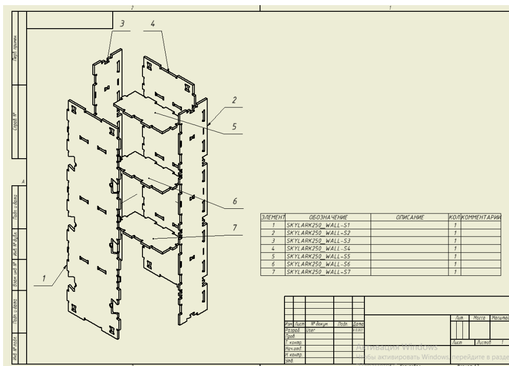
Рис. 2. Схема сборки стены
