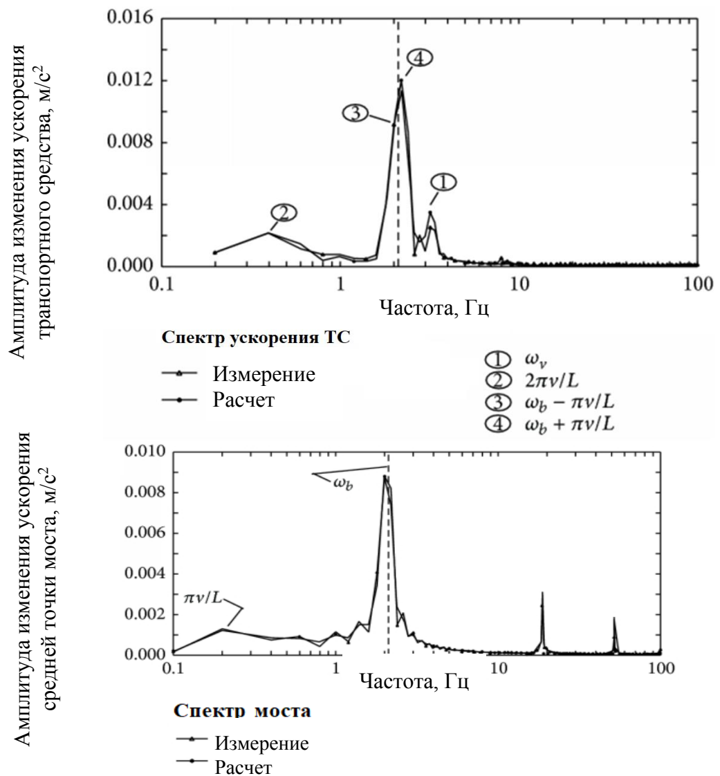
Спектр вертикального ускорения транспортного средства (вверху) и средней точки моста (внизу) при скорости движения транспортного средства v = 10 м/с
