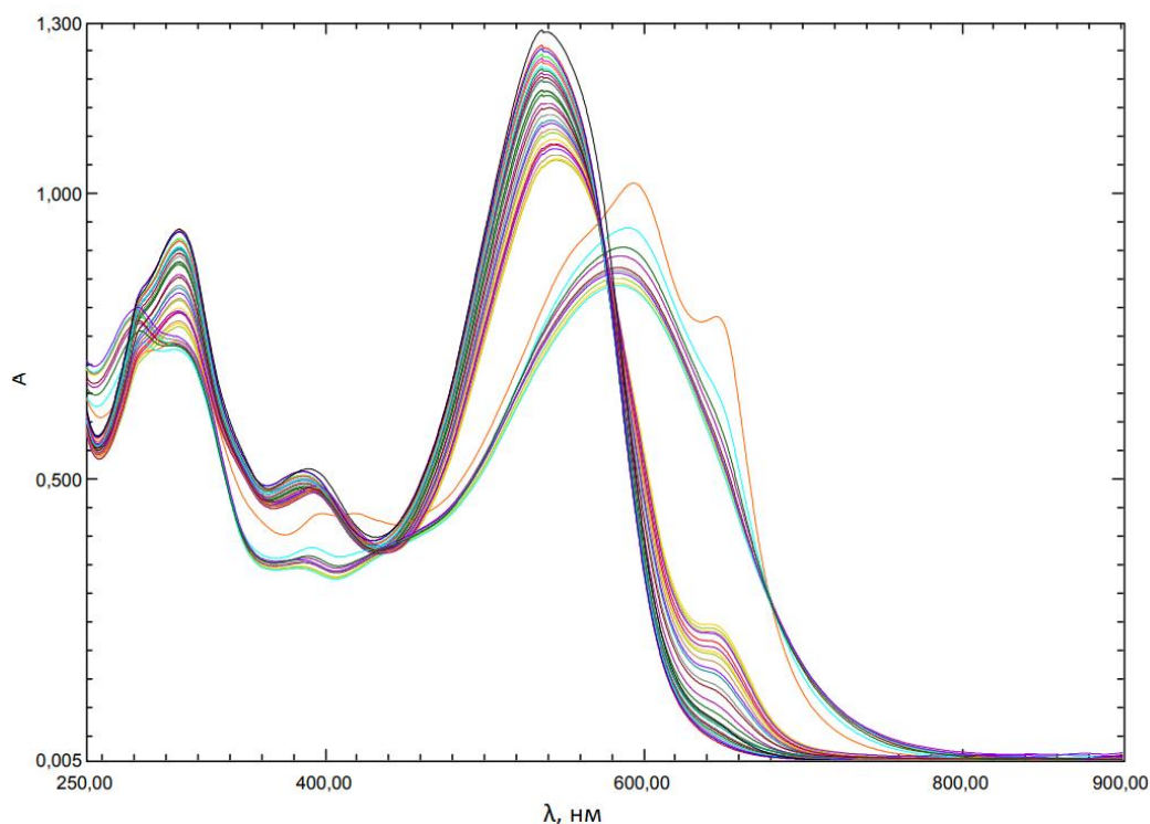
Рис. 1. Спектры поглощения арсенazo III при последовательном изменении рН от 3,4 до 12,9
