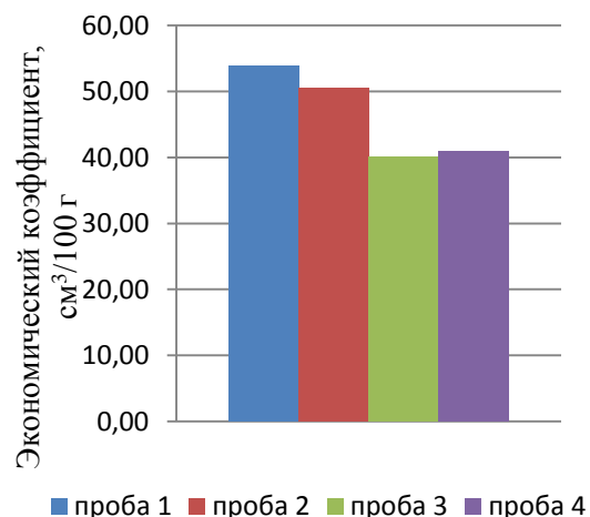
Рис. 5. Значения экономического коэффициента при 72-часовой ферментации
