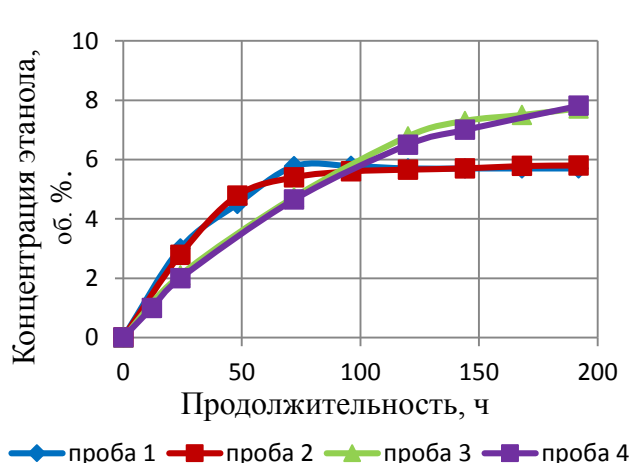
Рис. 4. Динамика биосинтеза этанола
