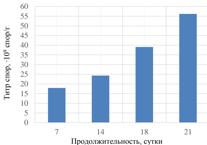
Рис. 2. Динамика конидиегенеза штамма К6-15 Trichodermas pp.
