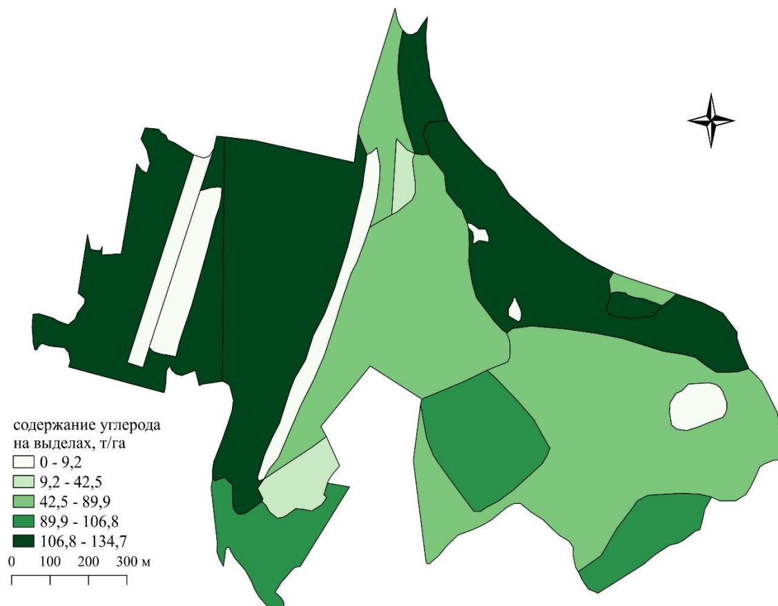
Карта распределения среднего содержания углерода на карбовом полигоне «Урал-Карбон (Коуровка)»
