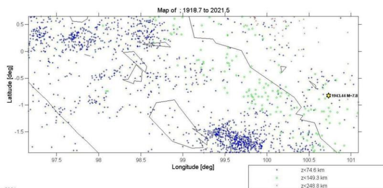
Gambar 2 Seismisitas gempa bumi yang terdampak di sekitar kota Pariaman
