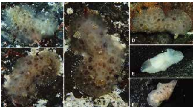
Fig. 3 - A) The Tayuva lilacina specimen in dorsal view. B) Right anterodorsal view. C) Dorsal view. D) The individual in extension. E) The ventral part of the body. F) The animal with the knurled appearance. (Photos by A. Lombardo). / A) L'esemplare di Tayuva lilacina in visione dorsale. B) Visione antero-dorsale destra. C) Visione dorsale. D) L'individuo in estensione. E) La parte ventrale del corpo. F) L'animale con l'aspetto zigrinato. (Foto di A. Lombardo).
