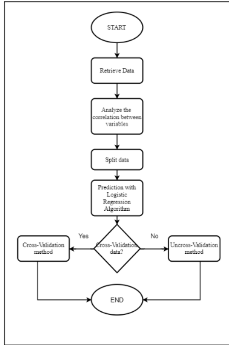
Fig. 1. Framework
