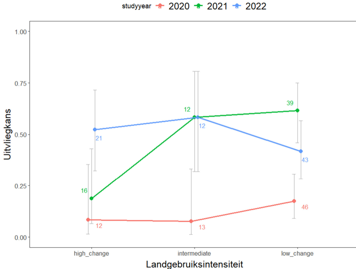
Figuur 3.1.14: De uitvlieggkans van met radiozenders gevolgde families in 2020 (rood), 2021 (groen) en 2022 (blauw) afhankelijk van de landgebruiksintensiteit van het weiland waar de kuikens uit het ei kwamen. Gemiddelden per landgebruiksintensiteit-categorie zijn uitgezet met 95% betrouwbaarheidsintervallen. Getallen naast de datapunten zijn de steekproefgroottes.
