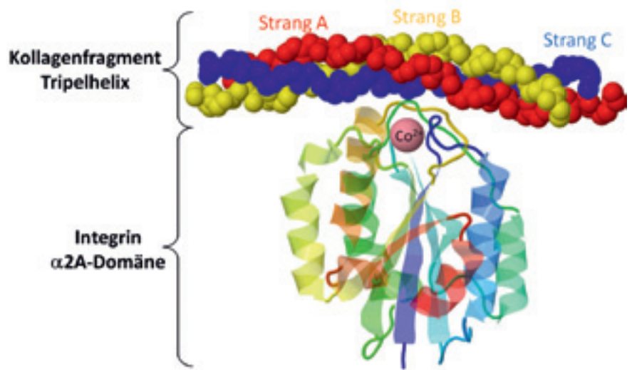
■ Abb. 2: Dreidimensionale Darstellung der tripelhelikalen Struktur eines Kollagenfragments: Strang A (rot), Strang B (gelb), Strang C (blau), gebunden an die \alpha 2A -Domäne des Integrins. Die Stränge sind ohne die Aminosäure-Seitenketten dargestellt.
