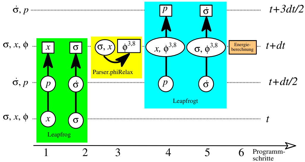
Abbildung 4.2: Berechnungsschema und -reihenfolge eines Simulationszeitschrittes. Die Namen “Leapfrog”, “Leapfrogt” und “Parser.phiRelax” beziehen sich auf die Subroutinen im Programm, die die entsprechenden Berechnungen ausführen. Rechtecke markieren Schreibvorgänge, Ovale und Kreise stehen für Lesevorgänge. Man bemerke, dass die Farbfelder ( \phi^a ) zwischen Zeitschritten nicht miteinander kommunizieren, weil das Gaußgesetz keine Zeitableitung enthält.
