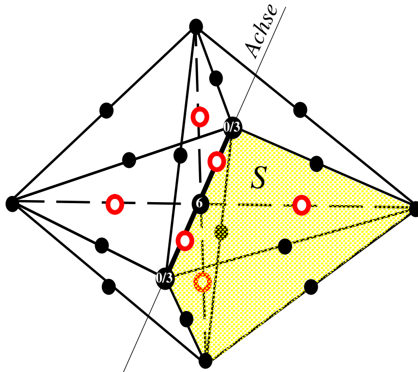
Abbildung 4.14: Dreidimensionale Verfeinerungszelle.
