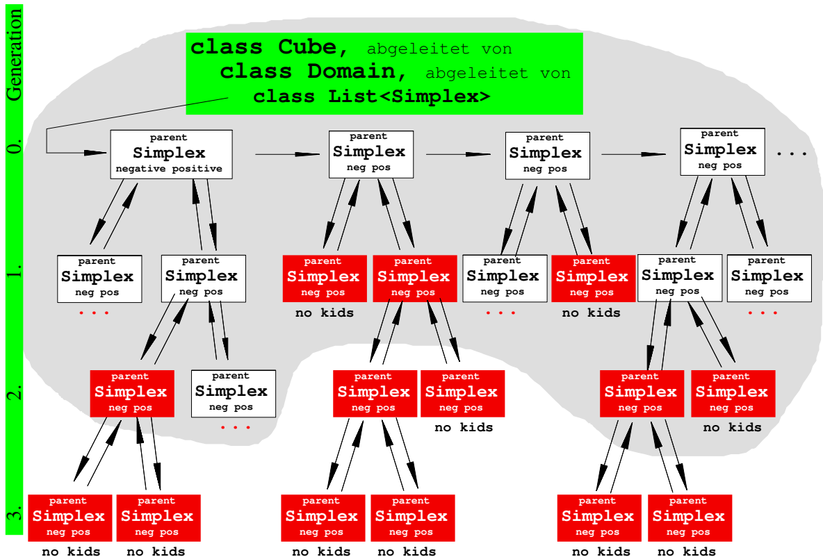
Abbildung 4.15: Der Simplexwald. Der grau schattierte Bereich deutet eine Sub-Wald-Struktur an, die mit Zäunen (Fences) erzeugt wird. Dabei sind in den rot (dunkel) schattierten Simplices alle Fences gesetzt (Erläuterungen dazu siehe Text). Der Nachbarschaftsgraph sowie die von den Simplices referenzierten Knoten, die auch Rückreferenzen auf ihre erzeugenden Simplices enthalten, sind hier aus Gründen der Übersichtlichkeit nicht dargestellt; diese Strukturen sind dem Graphen noch überlagert.
