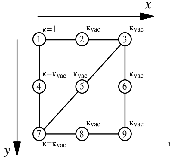
Abbildung 4.18: Das Simplexnetz \mathcal{T} mit zwei Simplexes bildet eine Partition des Einheitsquadrats. Die Knoten \{\vec{n}_1 \dots \vec{n}_9\} sind durch Kreise gekennzeichnet.
