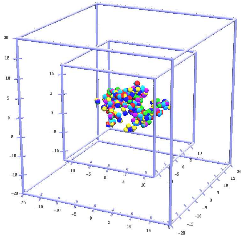
Abbildung 4.29: Unterschiedliche Gebietsgrößen für das Gitter des \sigma -Felds (kleiner Würfel) und das adaptive Knoten-/Simplexnetz des \phi^\alpha -Felds (großer Würfel). Da sich Farbladungen nur im \sigma -Feldgitter aufhalten können, bleiben sie immer in sicherem Abstand vom Rand des großen Würfels, jenseits dessen sich unphysikalische Spiegelladungen befinden.
