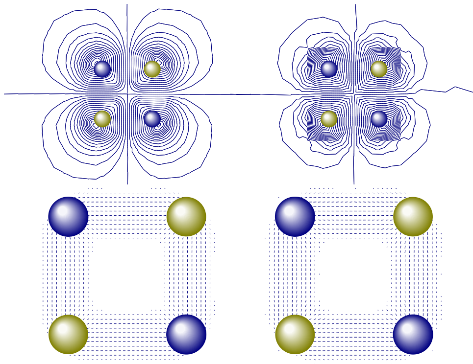
Abbildung 4.28: Qualität der Lösung des Testproblems (String-String-Konfiguration mit Stringlänge 4\text{ fm} und Stringabstand 4\text{ fm} ). In der linken Spalte ist die Lösungsfunktion \phi^8(\vec{x}) für den relativen Fehler r = 0.0001 der Lösung gezeigt, in der rechten Spalte das Gleiche für den relativen Fehler r = 0.01 . Auch die Lösung auf der rechten Seite ist noch qualitativ richtig und recht brauchbar.
