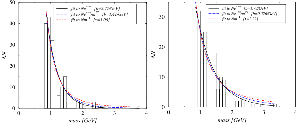
Abbildung 5.13: Massenverteilungen; der linke Graph gehört zum Bjorkenereignis, der rechte zum Full-Stopping-Ereignis.
