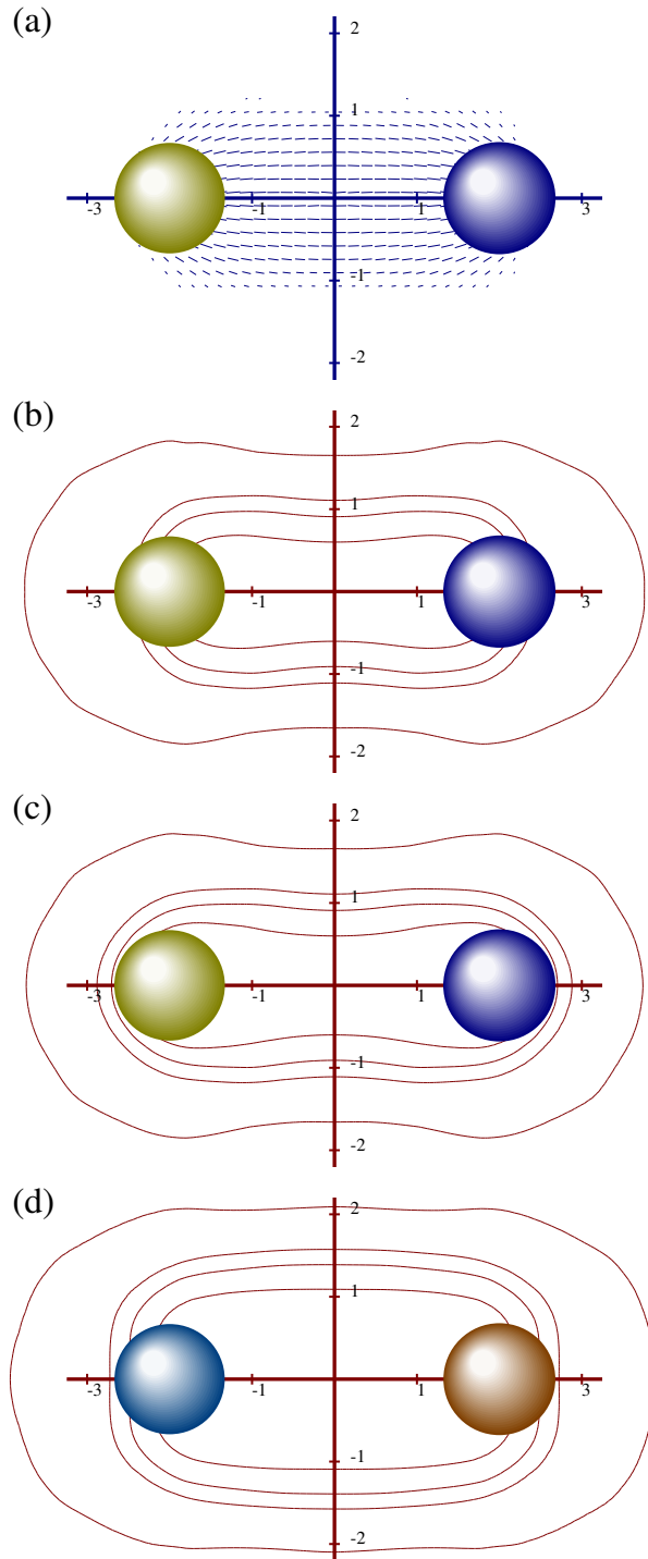
Abbildung 5.5: (a) Vektorfeld eines Quark-Antiquark-Flussschlauchs der Länge 4\text{ fm} . Die Energiedichte des gezeigten Vektorfeldes beträgt etwa 0.3\text{ GeV}/\text{fm}^3 . Die konkrete Farbwahl (blau-antiblaue) spielt für dieses Resultat keine Rolle. (b) \sigma -Feld des gleichen Flussschlauchs. (c) das gleiche Bild, modifiziert durch einen zusätzlichen skalaren Kopplungsterm (3.57) mit g_S = 8 . (d) \sigma -Feld eines gluonischen Strings. Äquipotentiallinien sind durch \sigma = 0\text{ fm}^{-1} , 0.1\text{ fm}^{-1} , 0.2\text{ fm}^{-1} , und 0.3\text{ fm}^{-1} definiert ( \sigma_{vac} \approx 0.31\text{ fm}^{-1} ). Die Striche auf den Achsen sind in Abständen von 1\text{ fm} gezeichnet.
