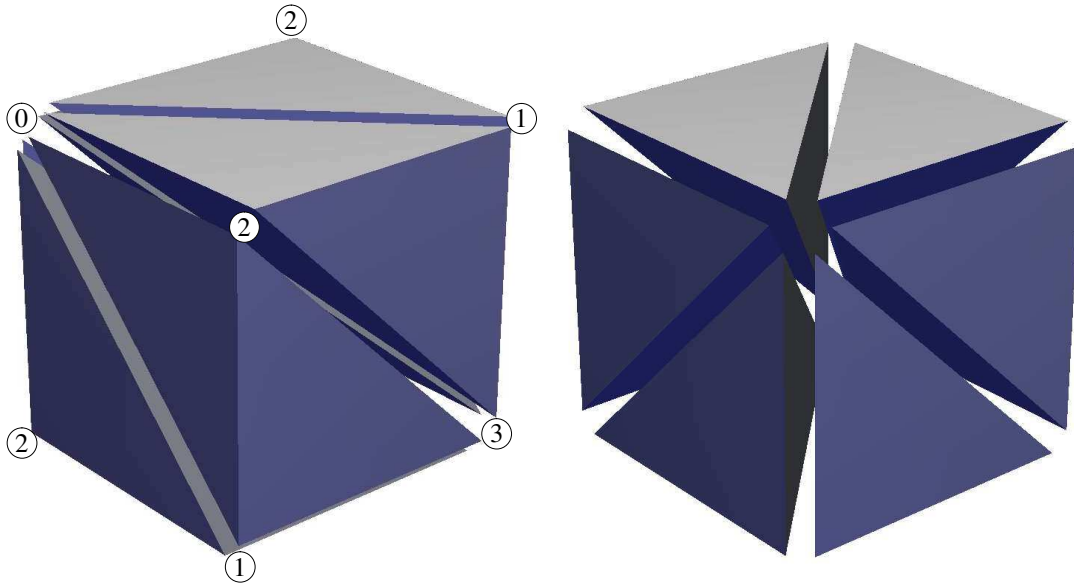
Abbildung 4.6: Partition eines würfelförmigen Gebiets in sechs kongruente Simplexes (‘‘Kuhnsimplex’’). Die Eckenknoten haben in jedem der Simplexes den gleichen Knotenindex, was nach dem Schema aus Abb. 4.5 auch für die Kantenknoten gilt.
