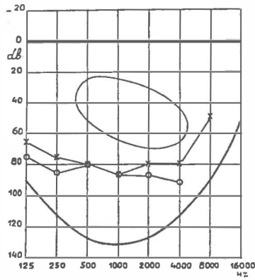
Fig. 19a. Drempelaudiogram bij een perceptiestoornis (komvormige curve).
