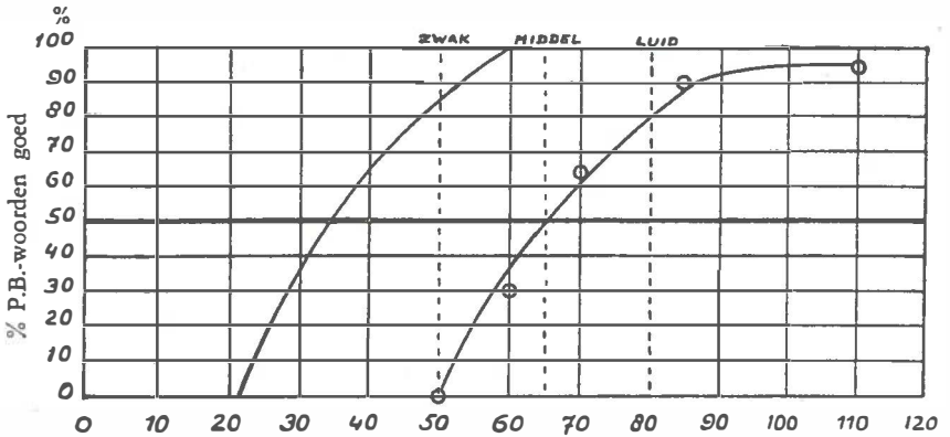
Fig. 17b. Spraakaudiogram bij een perceptiestoornis volgens fig. 17a.
