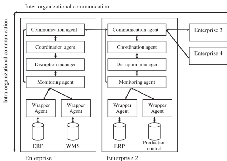
Εικόνα 25: Αρχιτεκτονική συστήματος MA διαχείρισης ρίσκου - Agents
