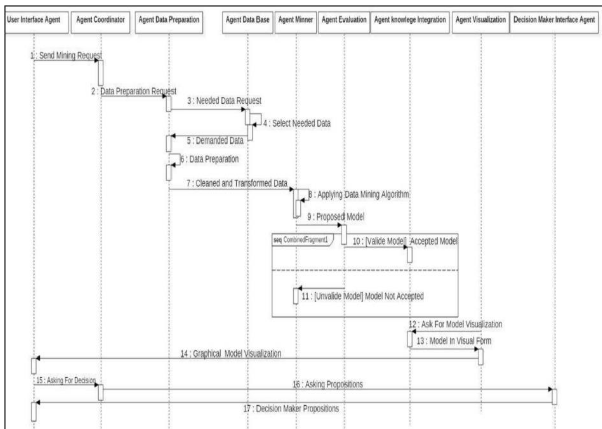
Εικόνα 4: Ροή λειτουργιών MADSS με χρήση KNN
