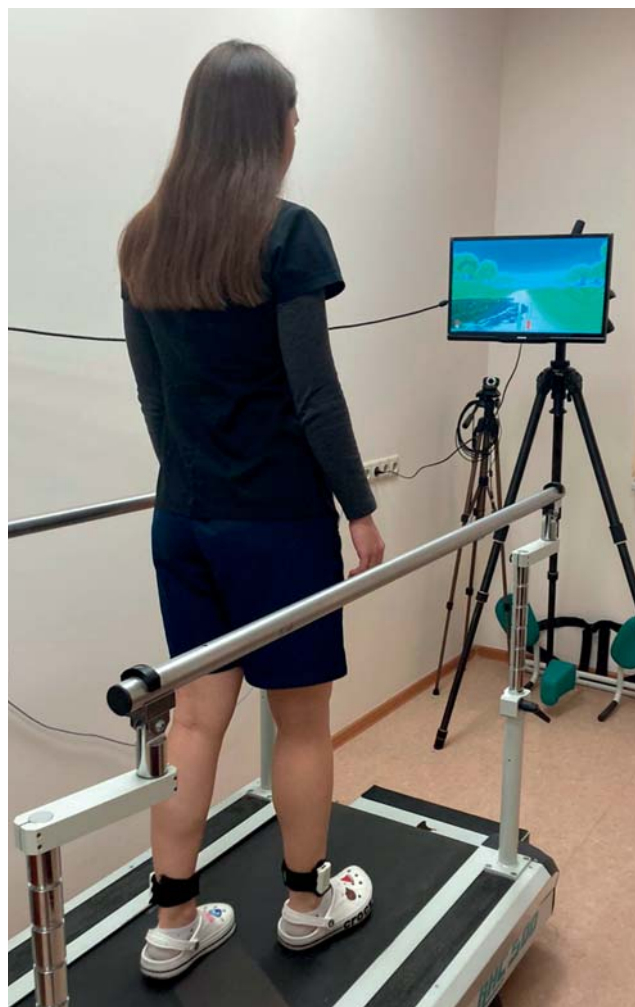
Рис. 1. Процесс тренировки.
