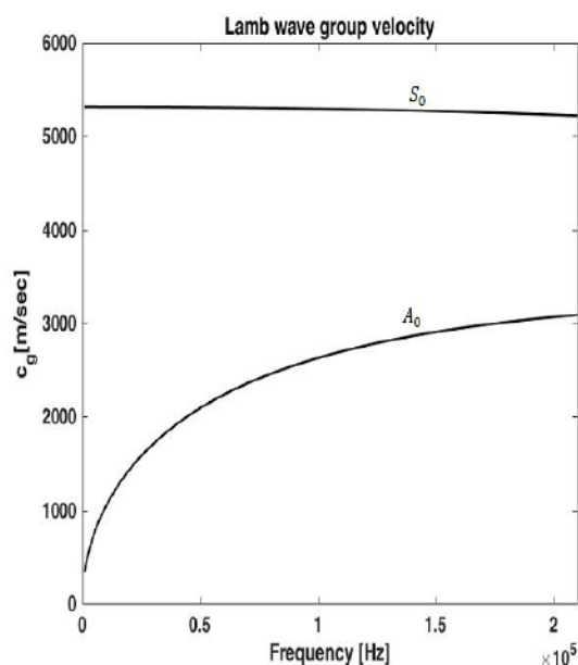
Fig. 2 Group velocity dispersion curve of the simulated aluminum plate شکل 2 نمودار پراکندگی سرعت گروه موج لمب در ورق آلومینیوم شبیه‌سازی شده
