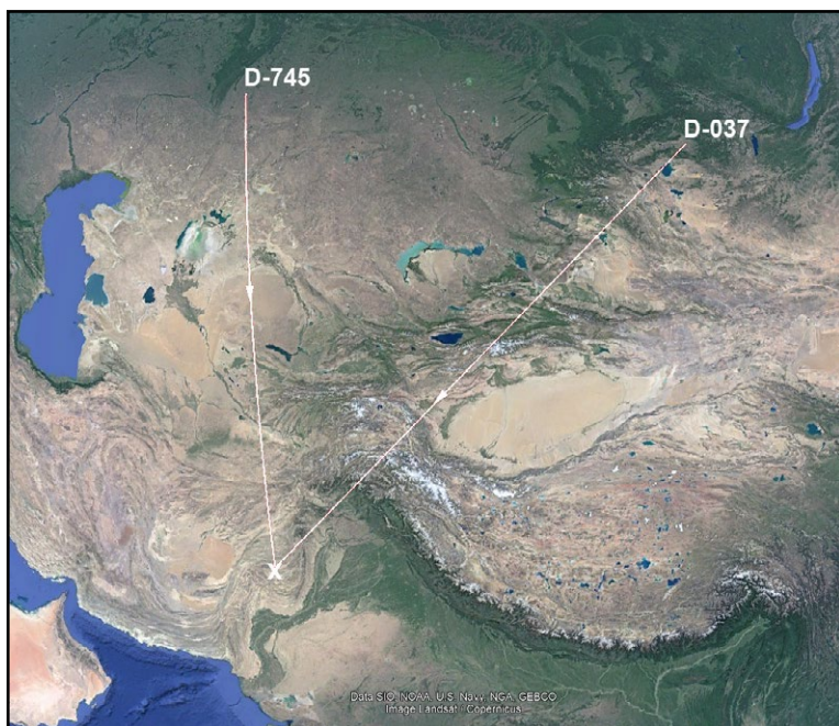
Рис. 1. Схема возврата колец от балобанов (Falco cherrug) «алтайского» фенотипа, выращенных в питомнике и выпущенных в природу на Южном Урале и в Алтае-Саянском регионе, которые были отловлены в Пакистане.
