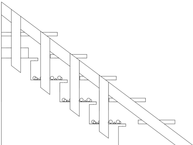
Figura 7.3.10. Esquema de la escalera diseñada en Crerev.
