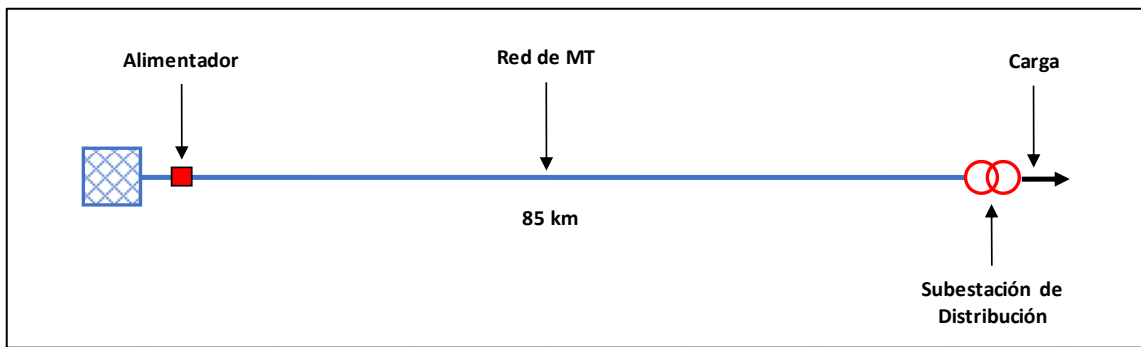
Figura 22: Red de media tensión simple
