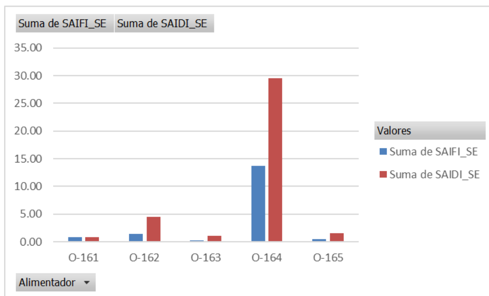
Figura 35: Resultados de los índices SAIFI y SAIDI por alimentador calculados mediante el Software microsoft 2016
