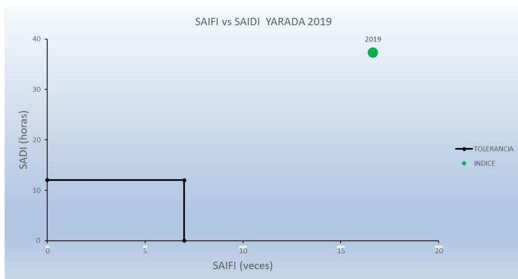
Figura 34: SAIFI y SAIDI del Sistema Eléctrico Yarada 2019
