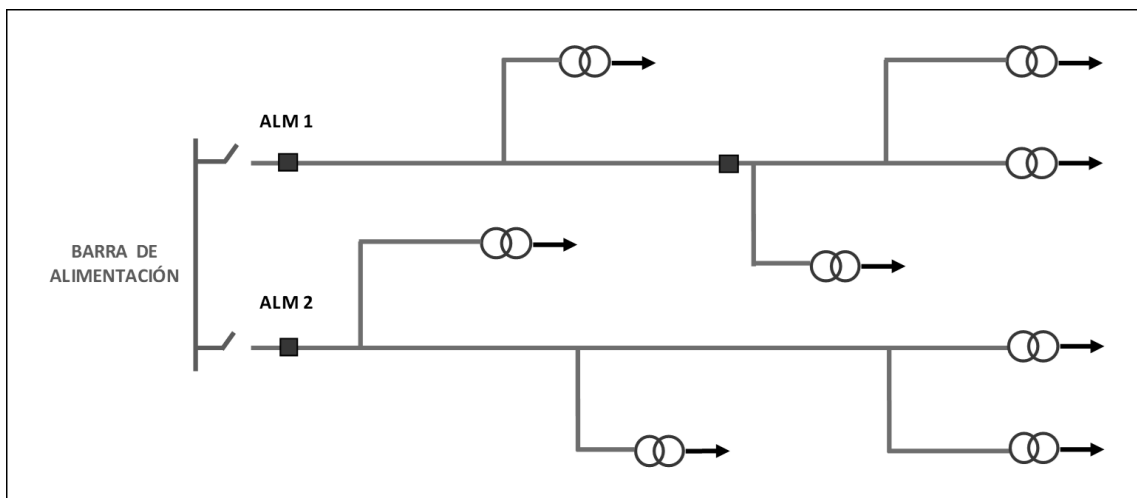
Figura 2: Sistema de distribución radial
