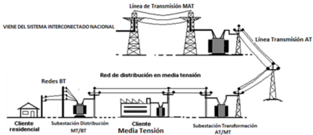
Figura 4: Sistema eléctrico de distribución
