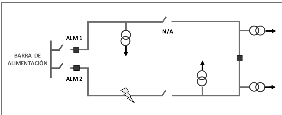
Figura 3: Sistema de distribución en anillo
