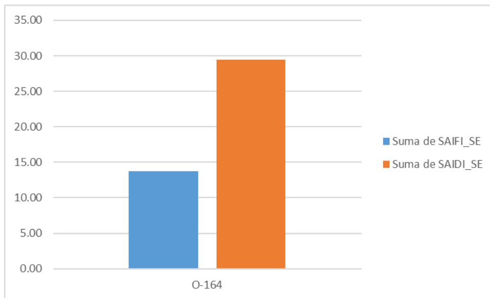
Figura 31: Modelo de falla para punto de seccionamiento O-164
