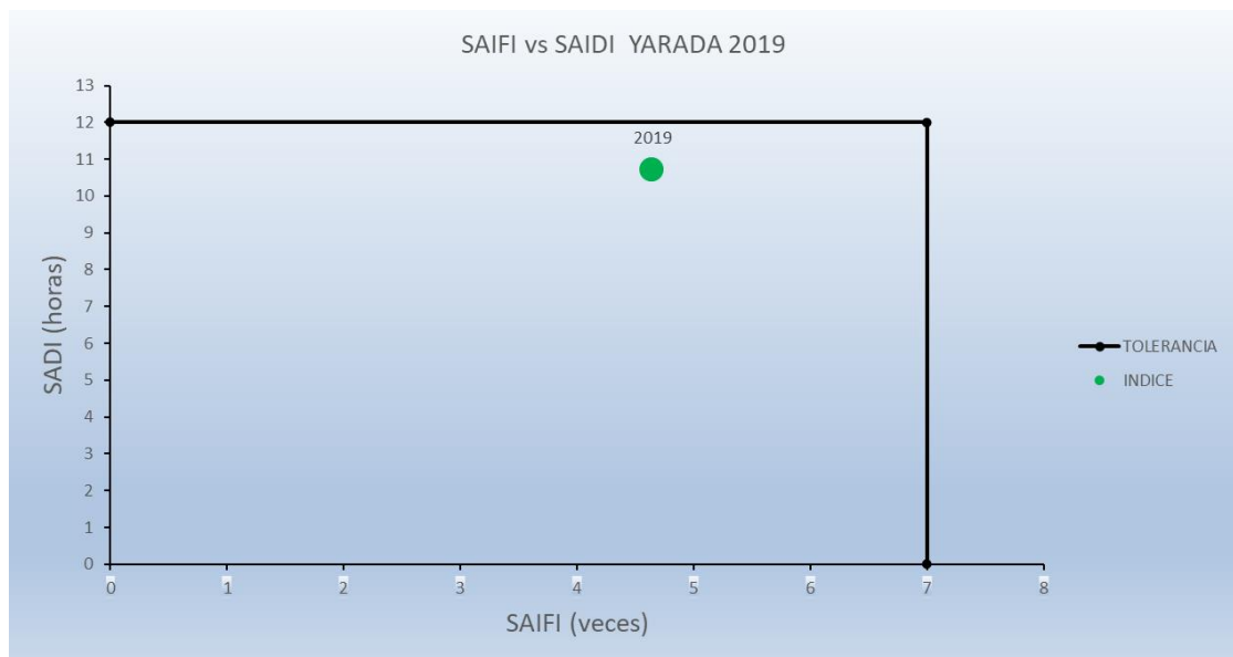
Figura 36: SAIFI y SAIDI del Sistema Eléctrico Yarada ubicación óptima.
