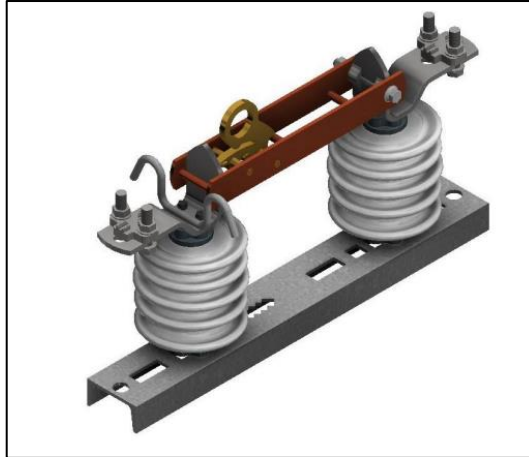
Figura 12: Seccionador monopolar tipo cuchilla
