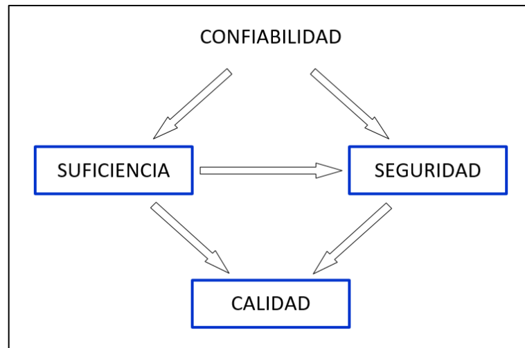
Figura 14: Atributos del sistema eléctrico relacionados a la confiabilidad
