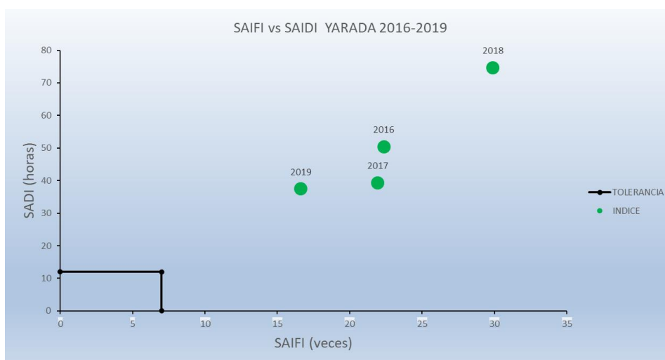
Figura 33: SAIFI y SAIDI del Sistema Eléctrico Yarada 2016-2019
