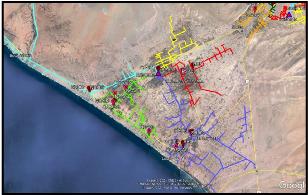
Figura 30: Sectorización de redes de distribución.
