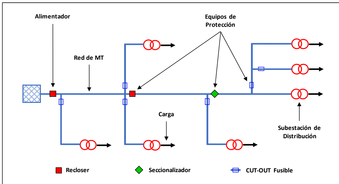
Figura 5: Alimentador en media tensión (Elaborado por mi persona)
