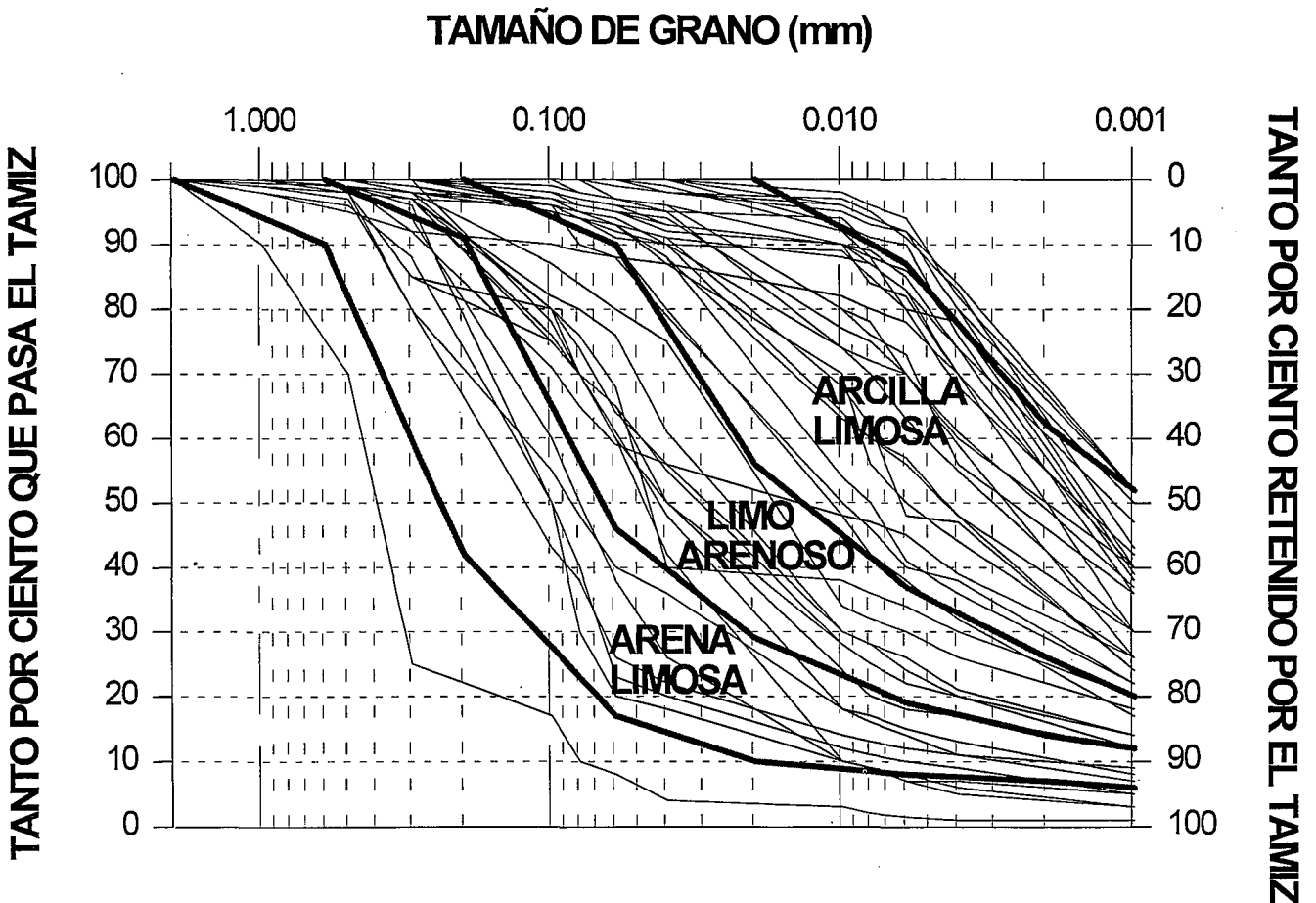
Fig. 4.- Curvas granulométricas.
