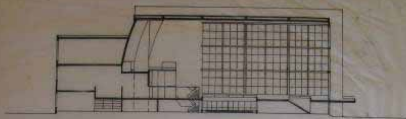
COUPE LONGITUDINALE
