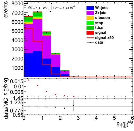
(b) DeltaEtaSignalJets
