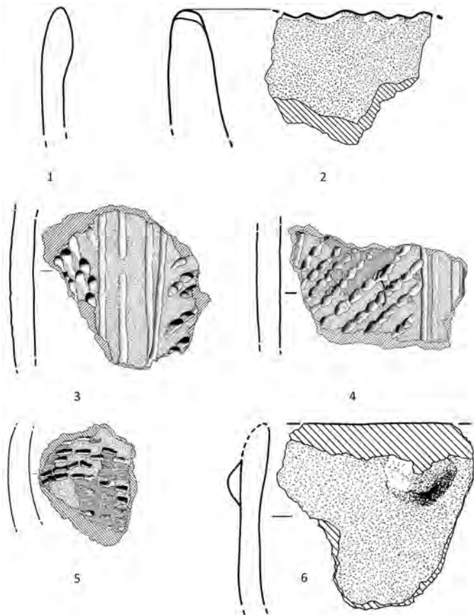
Fig. 6 Bazel (prov. Oost-Vlaanderen/B). Bone tempered pottery. – (Drawings M. Van Meneen). – Scale 1:4.
