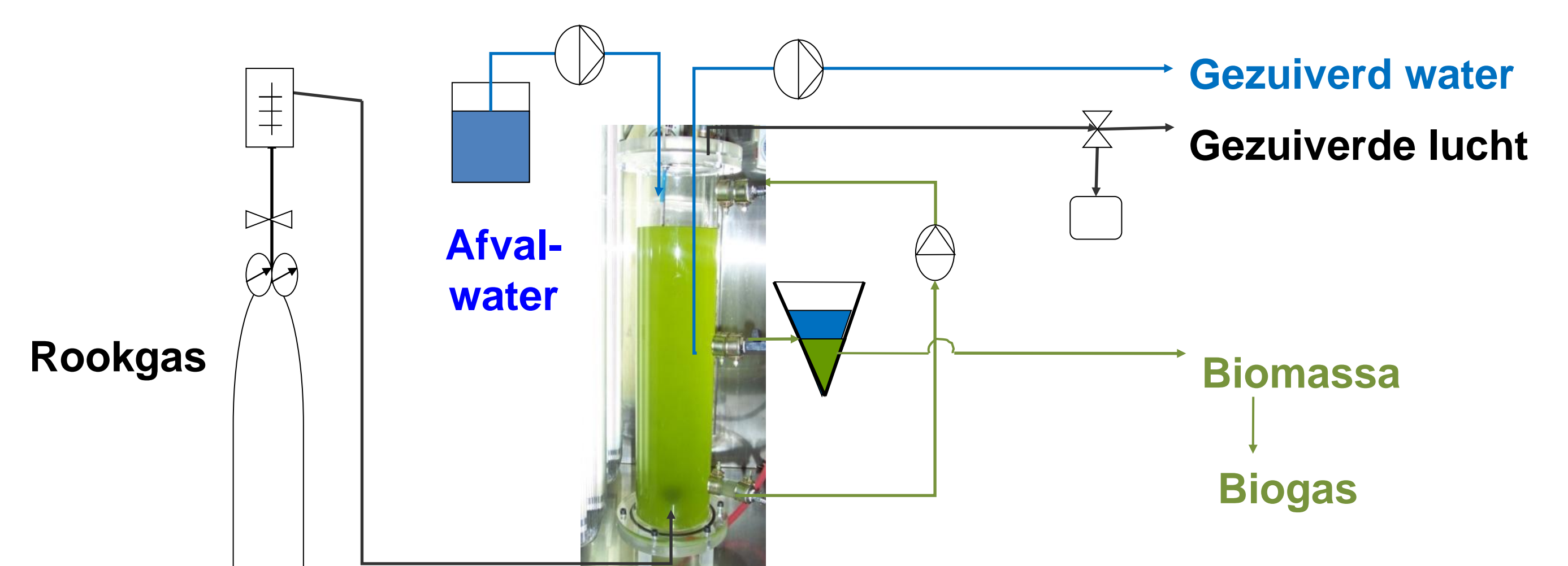
Schema opstelling rookgaszuivering met microalgen
