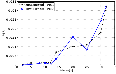
Fig. 18. PER indoor
