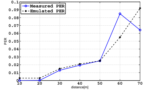
Fig. 19. PER outdoor
