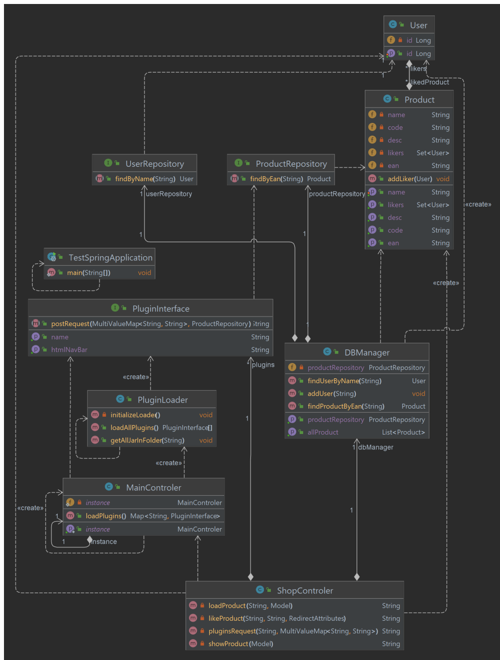
FIGURE 5.1 – Diagramme de classes de la plateforme web Shop
