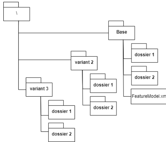
FIGURE 4.6 – Arborescence à respecter pour une ligne de produits
