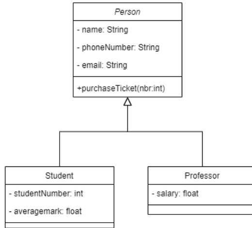
FIGURE 2.7 – Diagramme montrant l’héritage de classes
