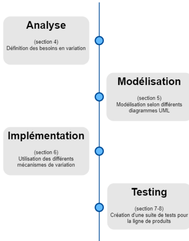
FIGURE 1.1 – Les différentes étapes de développement d'une ligne de produits
