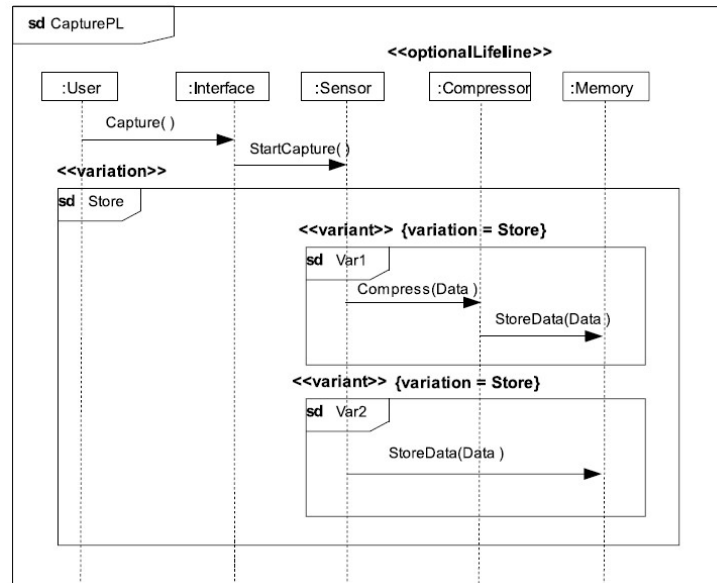
FIGURE 2.4 – Diagramme de séquence
