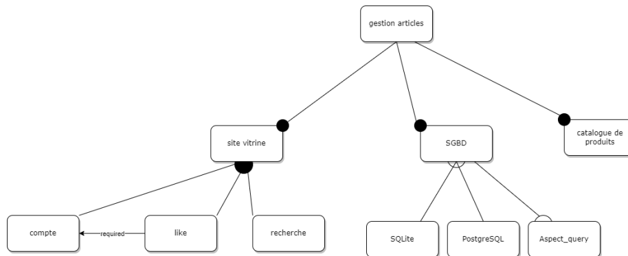
FIGURE 5.2 – Diagramme de features de la plateforme web Shop
