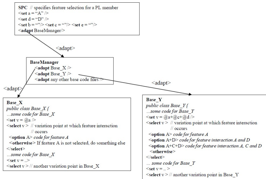
FIGURE 2.9 – illustration du fonctionnement de XVCL
