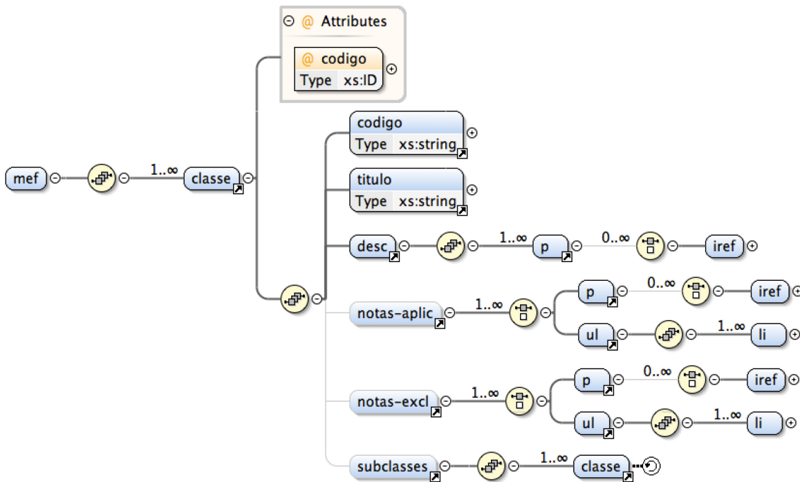
FIGURA 1: XML SCHEMA DA MEF- MEFML
