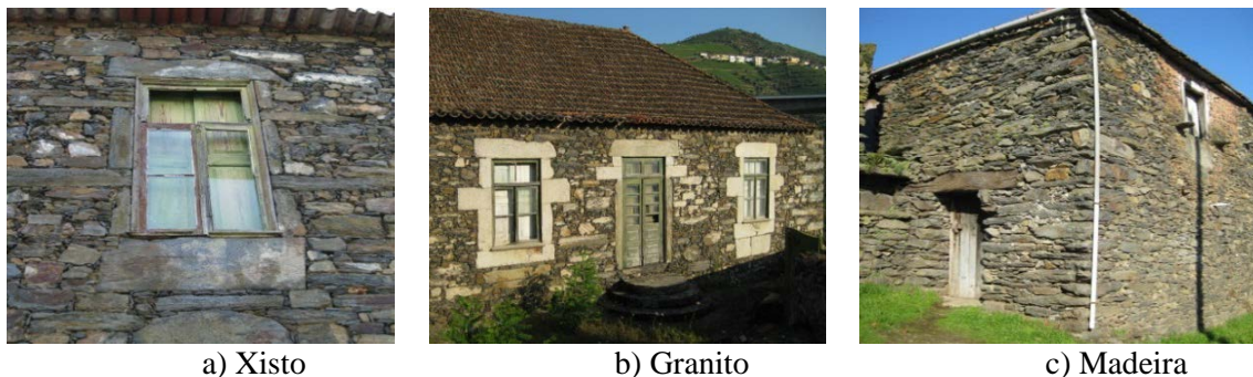
Figura 7: Materiais aplicados na construção de elementos de padieira, de ombreira e de peitoril
