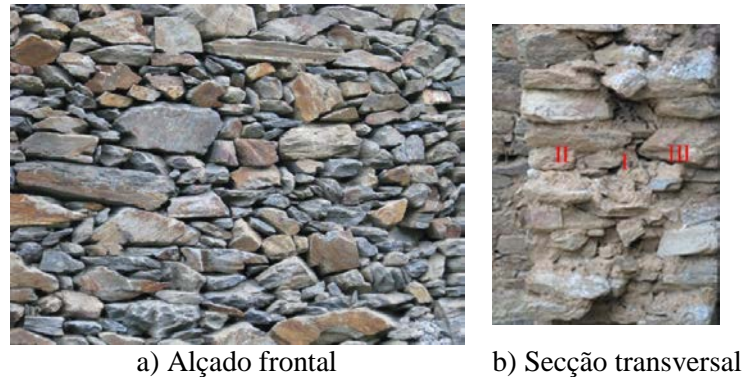
Figura 2: Detalhes construtivos de paredes de alvenaria de pedra de xisto
