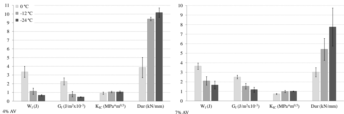
Figura 5. Mecanismos de fratura a temperaturas baixas.
