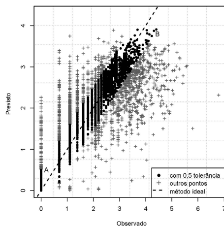
Figura 3 - RSC do modelo RF
