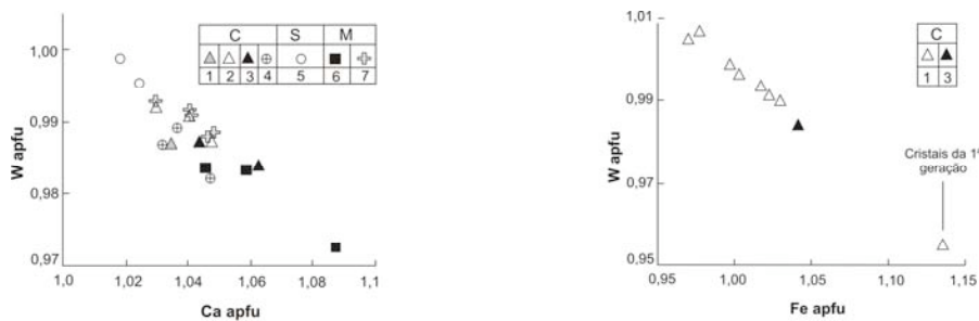
Fig. 3 – Composições de tungstos presentes em associações de Covas, Serro e Monteiro. Nota: as composições de volframites de Covas incluem pseudomorfoses e cristais da 1ª geração. Legenda: C- composições de Covas (fácies com sulfuretos maciços-2 e 4, grossularitos - 1 e metasomatitos - 3); S- composições do Serro (rochas calcossilicatadas -5 ); M – composições do Monteiro. (anfíbolitos - 6 e fácies peri-anfíbolicas leucocratas - 7).
