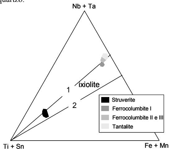
Fig. 4: Projecção dos conteúdos catiônicos dos óxidos de Ti-Nb-Ta no diagrama triangular Ti + Sn - Nb + Ta - Fe + Mn. Linhas de substituição: 1 - 3(Ti, Sn) 4+ - (Fe, Mn) 2+ 2(Nb, Ta) 5+ ; 2 - 2(Ti, Sn) 4+ - (Fe 3+ , Mn) (Nb, Ta) 5+ .
