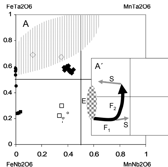
Fig. 3: Projecção das composições da struverite, columbite-tantalite e microlite no diagrama columbite/tantalite – tapiolite (A). A'- tendências de fraccionação e substituição mineralógicas ajustadas à localização paragenética. Símbolos: ● - struverite; ■ - Fe-columbite I; □ - Fe-columbite II; Δ - Fe-columbite III; ◆ - tantalite; ◇ - microlite. E - equilíbrio struverite-ferrocolumbite I; F1 - fraccionação paragenética primária; F2 - fraccionação cristalina primária; S - tendências de substituição.
