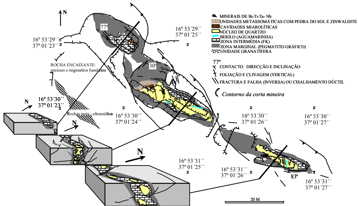
Fig. 1: Área de prospecção de Melatube (estrutura interna) – esboço simplificado e reconstituição 3d não isométrica do grupo pegmatítico; as coordenadas geográficas são indicadas para posicionamento global.
