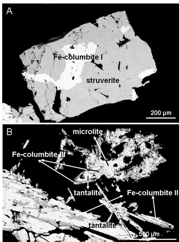
Fig. 2: Imagens MEV – ER dos intercrescimentos e modos de contacto entre os minerais de Ti-Nb-Ta. A- geometria compósita de ferrocolumbite I e struverite; B- intercrescimentos de ferrocolumbite II e tantalite; zonamento oscilatório e textura de intercrescimento vermiforme de ferrocolumbite III e tantalite; aspecto da substituição dos Nb-tantalatos por microlite.
