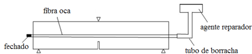
Figura 4 – Diagrama esquemático do sistema de abastecimento externo contendo o agente de reparação, baseado na descrição de Mishashi e Joseph (Wu et al., 2012)
