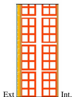
Figura 6. Solução Fach. 5 - Rebocos Isolantes
