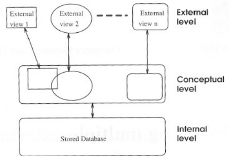
Fig. 1. ANSI/SPARC architecture.
