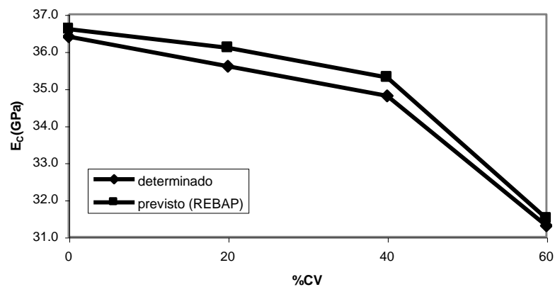
Figura 2 - Módulo de elasticidade dos betões ensaiados
