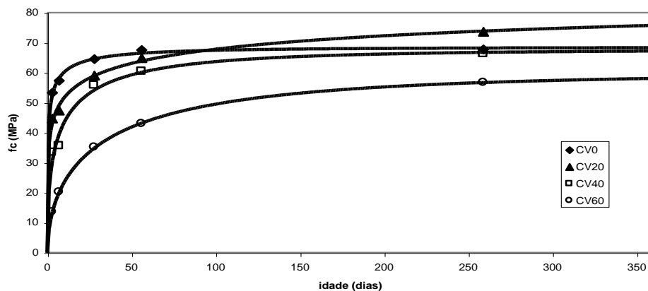
Figura 1 – Evolução da resistência ao longo do tempo.
