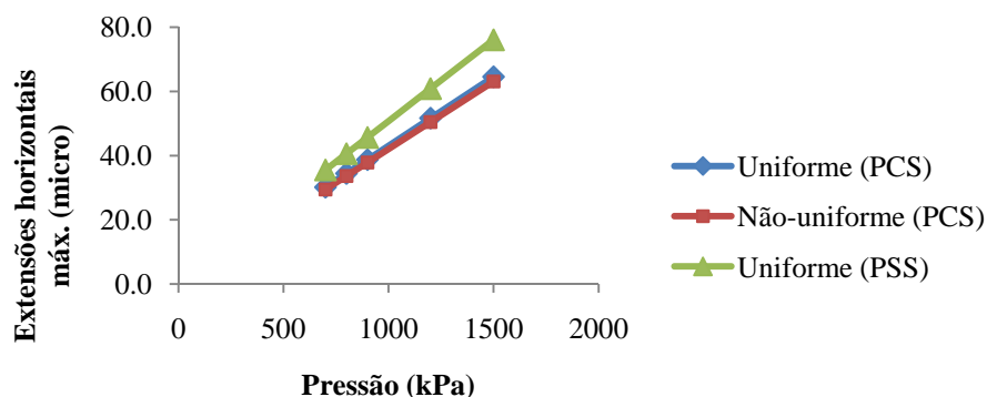
Figura 14. Extensão horizontal localizada na base da última cada betuminosa para diferentes intensidades e configuração de pressão de enchimento
