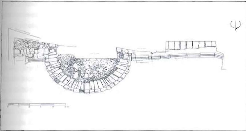
Fig. 5 – Desenho do torreão da muralha do Baixa Império, estrutura que se sobrepôs, sem inutilizar a conduta de água limpa. (Arquivo UAUM)
