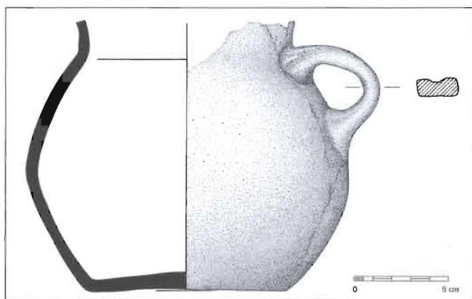
Fig. 10 – Banhos castrejos da ECFB: desenho do vaso encontrado na base da estrutura. (Arquivo MDDS)
