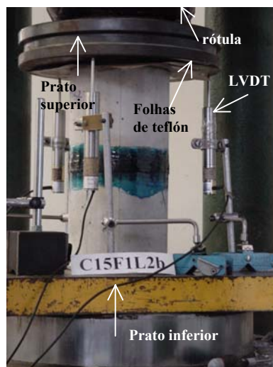
Figura 9 – Posição dos três LVDTs.
