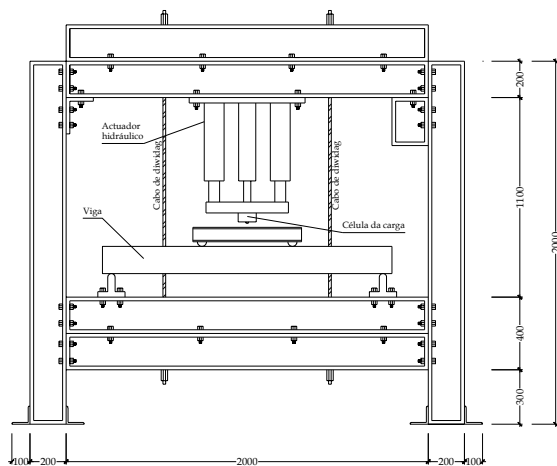
Fig. 2 – Sistema de ensaio das vigas
