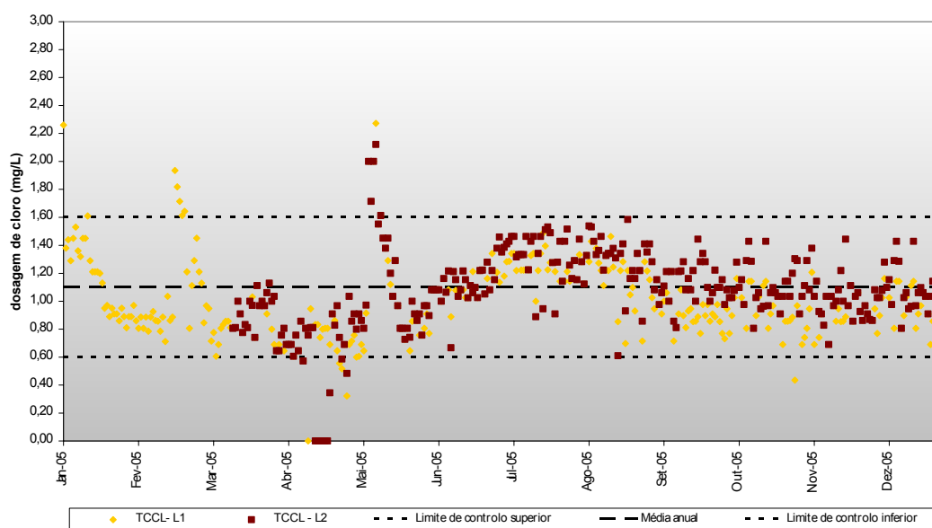
Figura 3 Variação de dosagem de cloro na desinfecção – PCC 5
