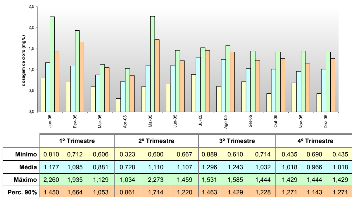
Figura 4 Análise estatística de dosagem de cloro na desinfecção – PCC 5
