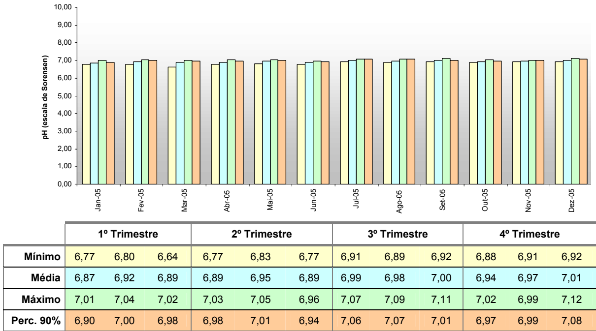
Figura 6 Análise estatística de pH na desinfeção – PCC 5
