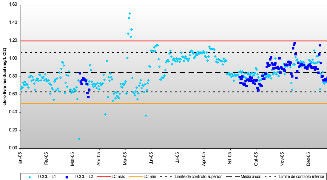
Figura 7 Variação de cloro livre residual na desinfeção – PCC 5
