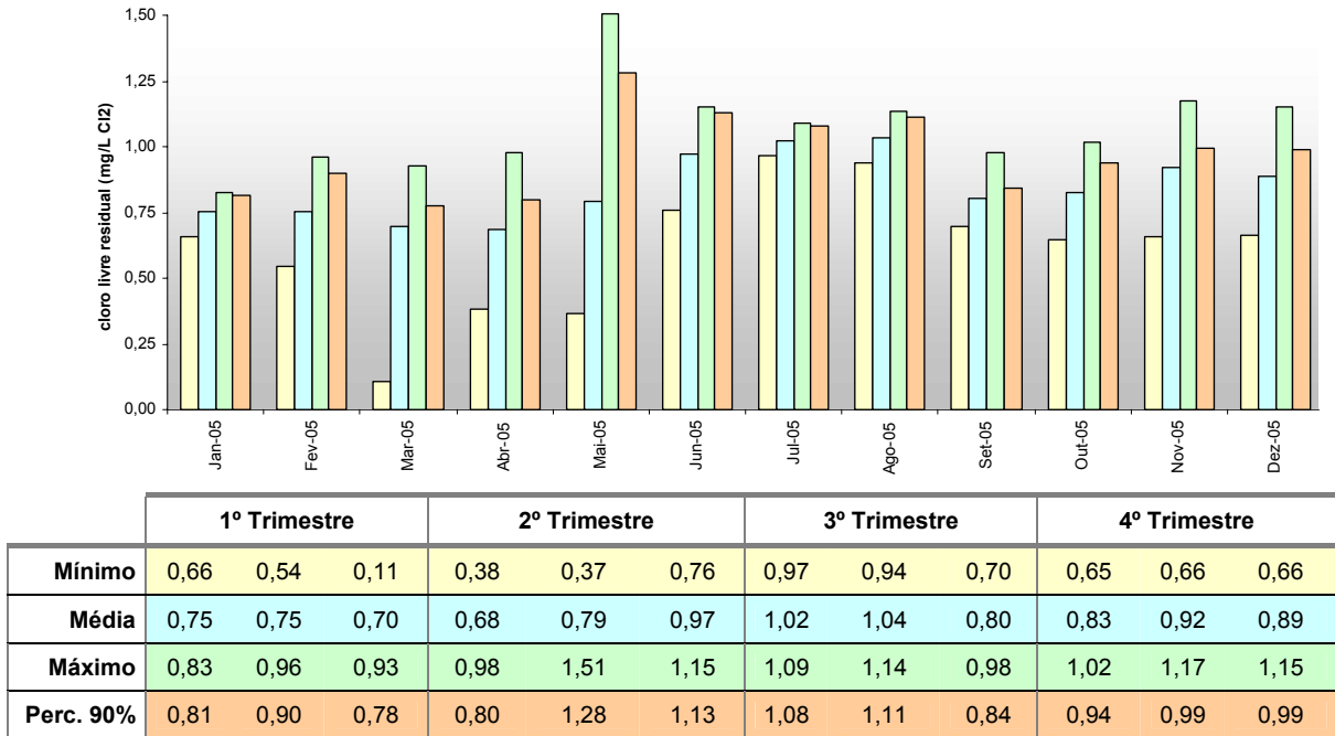
Figura 8 Análise estatística de cloro livre residual na desinfecção – PCC 5
