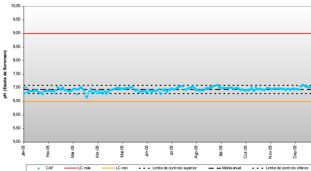
Figura 5 Variação de pH na desinfecção – PCC 5
