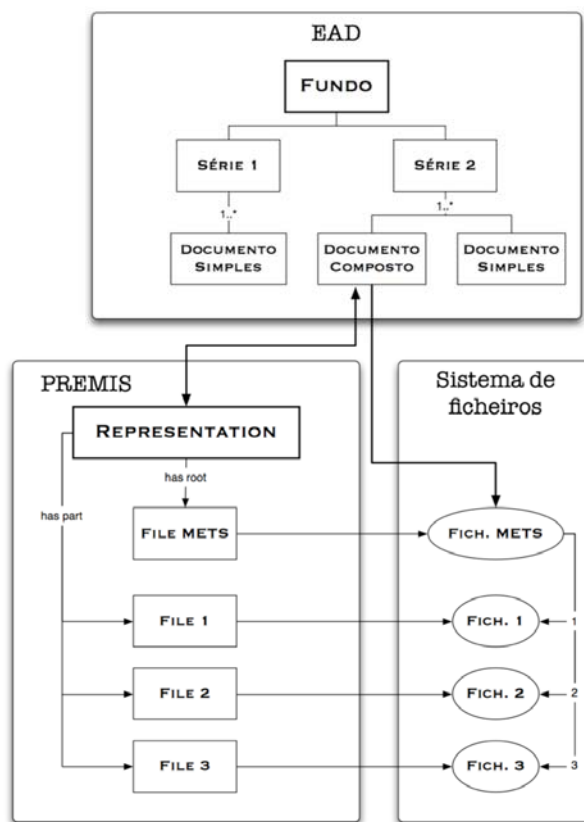
Figura 5 - Esquema completo (excepto NISO Z39.87)
