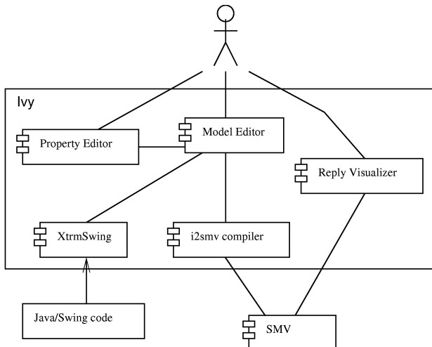
Figura 3 - Arquitetura da ferramenta IVY
