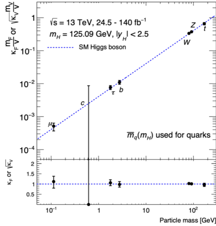
Figure 8.10: De koppingssterktemodificatoren \kappa_f m_f / v en \sqrt{\kappa_V} m_V / v als functie van de massa's van de fermionen m_f en vectorbosen m_V . De limiet op de koppingssterktemodificator \kappa_c , overeenkomend met 68% CL, uit de VH(\rightarrow c\bar{c}) -analyse wordt geïllustreerd met de andere koppingssterktemodificatoren die zijn verkregen uit een gecombineerde fit van analyses van het Higgs-deeltje uitgevoerd door de ATLAS-collaboratie [11].
