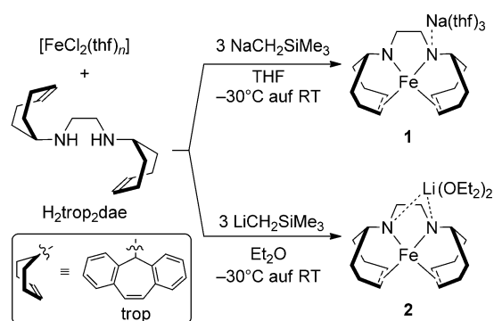
Schema 1. Synthese der Komplexe 1 und 2 ausgehend von [FeCl_2(thf)_n] ; 1 : n = 1.5 ; 2 : n = 0 .
